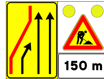
Figura 399/b Art. 39 Presegnale di cantiere mobile
