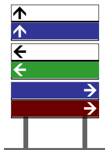
Figura 253 Art. 128 Gruppo segnaletico unitario urbano monofilare
